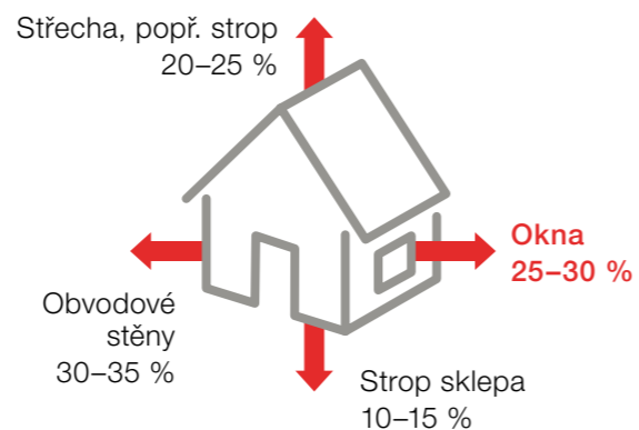
Obr.: Příklad tepelných ztrát způsobených prostupem tepla u běžného rodinného domu
